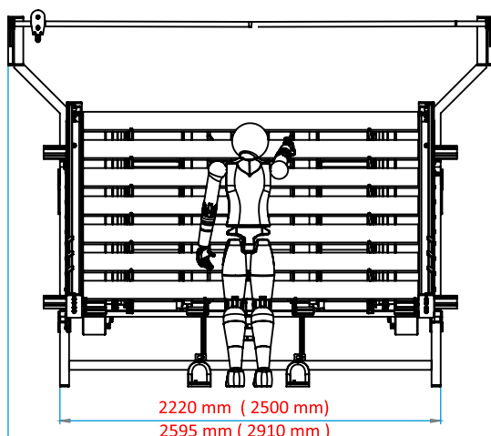
Wymiary stołu HS1800, w nawiasach dla modelu HS2200
