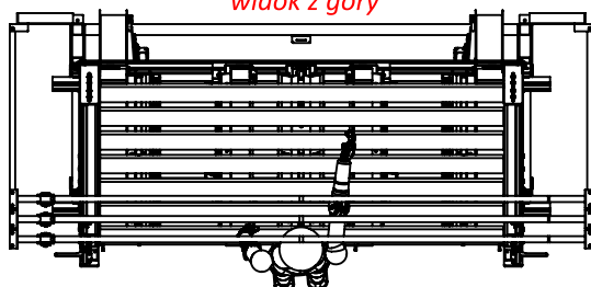
Wymiary stołu HS1800, w nawiasach dla modelu HS2200
